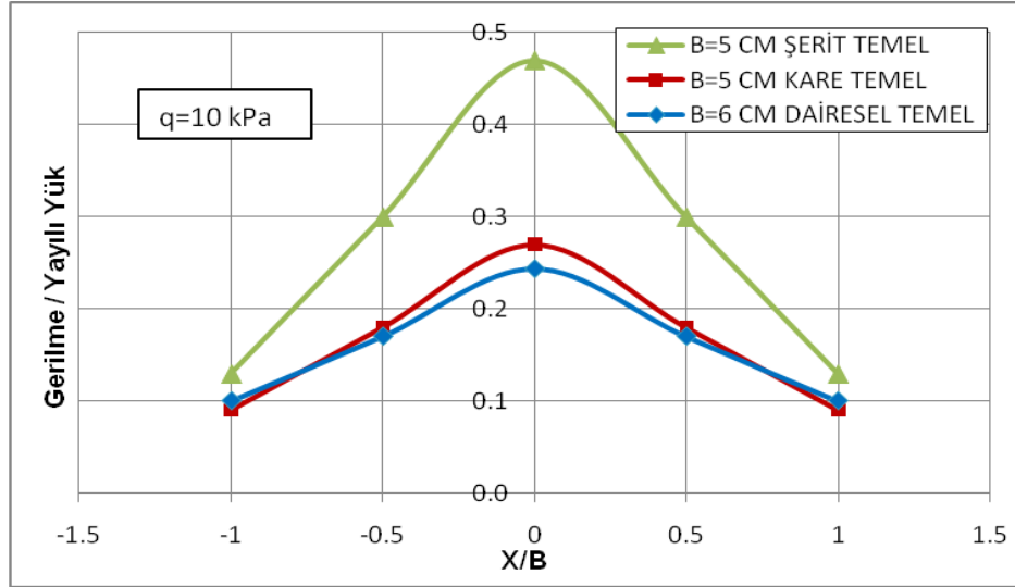
Şekil 14. Farklı Geometrilere Ait Temellerde Şekil Etkisi
