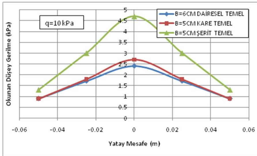
Şekil 13. q=10 kPa Değerinde Şekil Etkisi
