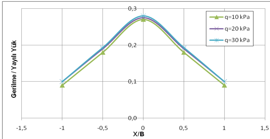
Şekil 11. Kare Temelde Yükün Etkisi ( B=5\text{ cm} )
