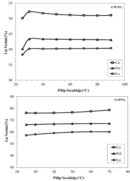
Şekil 9. H 2 SO 4 (%35 PKO, 220 dk liç süresi ve 400 kg/ton H 2 SO 4 ) (a) ve HNO 3 (%35 PKO, 120 dk liç süresi ve 400 kg/ton HNO 3 ) (b) liçinde NTE çözünme verimlerinin pülöp sıcaklığına göre değişim sonuçları
