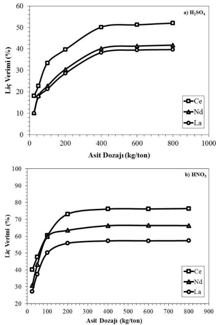
Şekil 8. H 2 SO 4 (%35 PKO, 220 dk liç süresi, ve 25°C pülöp sıcaklığı) (a) ve HNO 3 (%35 PKO, 120 dk liç süresi, ve 25°C pülöp sıcaklığı) (b) liçinde NTE çözünme verimlerinin asit dozajına göre değişim sonuçları
