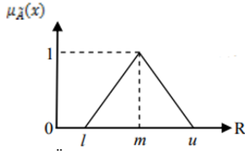
Şekil 1. Üçgensel bulanık sayı
