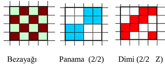
Şekil 1. Kumaş numunelerinin örgü tipleri
