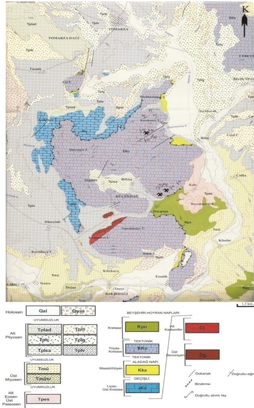
Şekil 2. Çalışma alanı jeoloji haritası [1].
