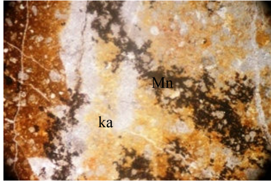
Şekil 5b. Yankayaç ince kesit görünümü, mikrokristalin kalsit kristalleri (ka) ve manganiz mineralleri (Mn), çift nikol
