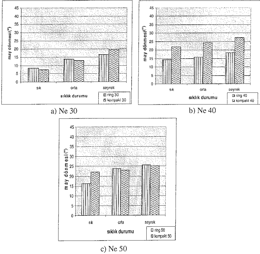
Şekil 4. Farklı iplik türü ve iplik numaraları için kumaş sıklığı-may dönmesi ilişkisi (kuru relakse)
