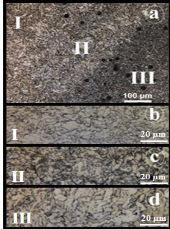
Şekil 3. a) Kaynak metali – ITAB – Ana metal mikroyapı görüntüsü, b) Ana metal mikroyapı görüntüsü, c) ITAB mikroyapı görüntüsü, d) Kaynak metali mikroyapı görüntüsü
