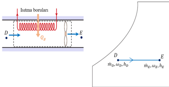
Şekil 4. Son ısıtma işleminin psikometrik diyagramda gösterimi
