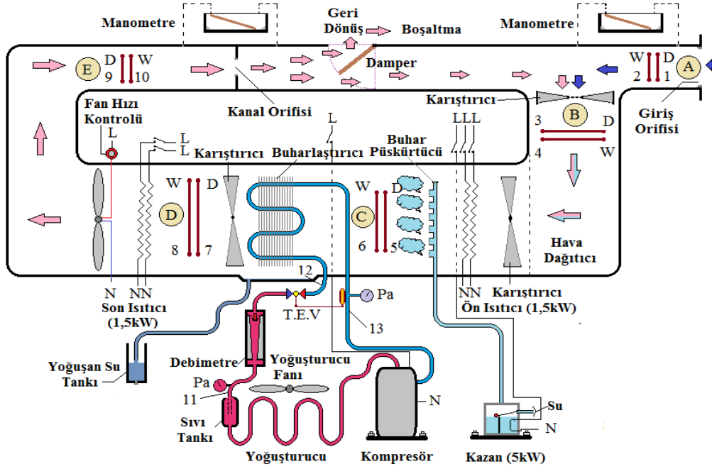
Şekil 1. Geri dönüş havalı iklimlendirme santrali
