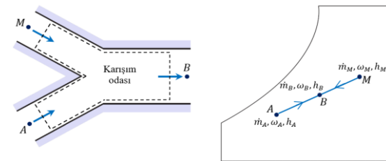
Şekil 2. Adyabatik karışma işleminin psikometrik diyagramda gösterimi
