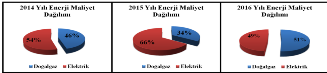
Şekil 4. 2014-2016 yıllarında KMÜ'ne ait tüketilen enerjinin maliyet dağılımı
