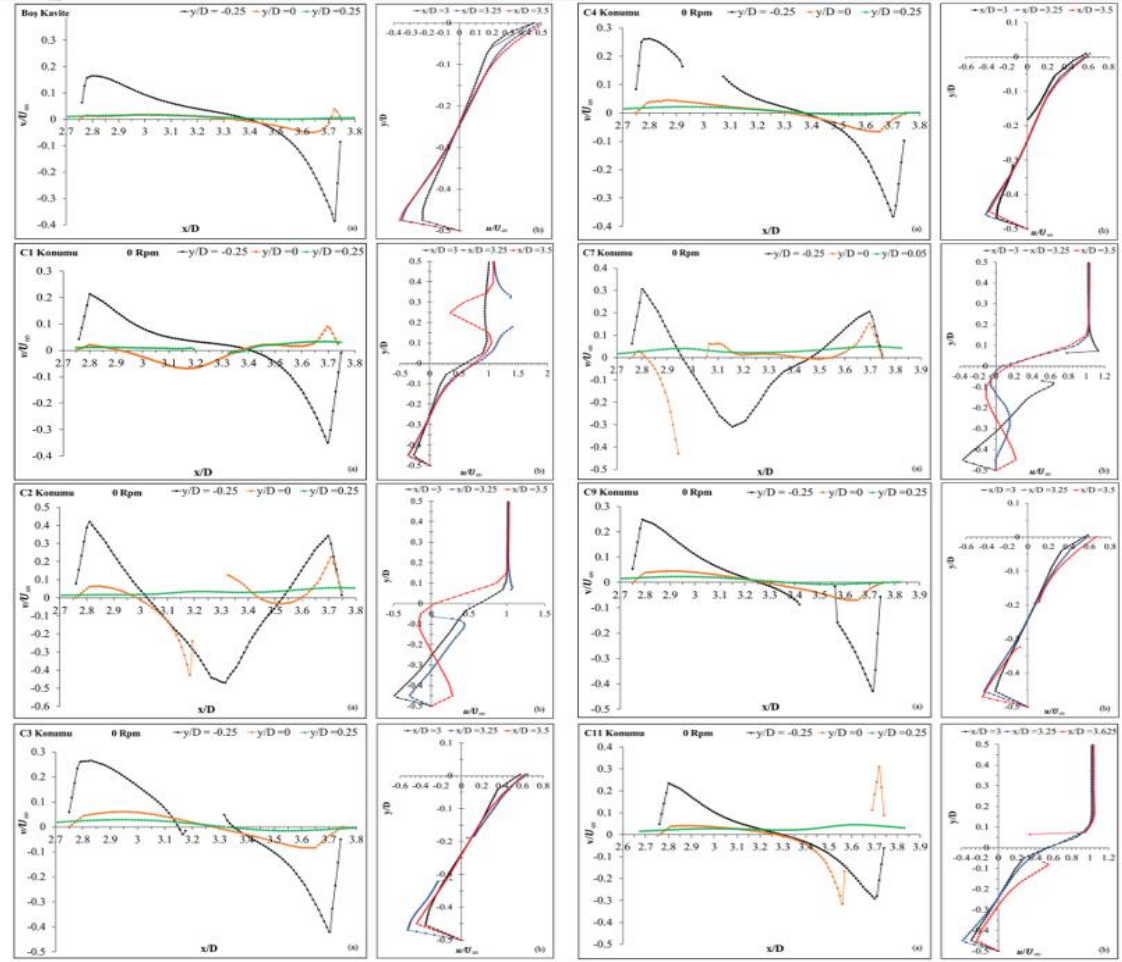
a) Akışa dik doğrultudaki boyutsuz hız profili b) Akış doğrultusundaki boyutsuz hız profili Şekil 6. Değişen silindir konumlarına göre boyutsuz hız profilleri
