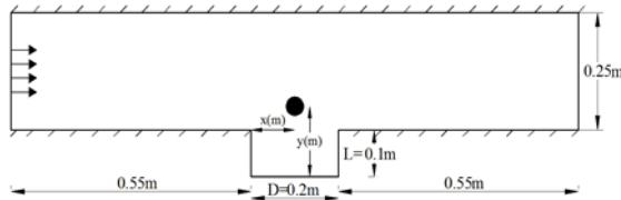
Şekil 1. Kavitenin şematik gösterimi ve model ölçüleri
