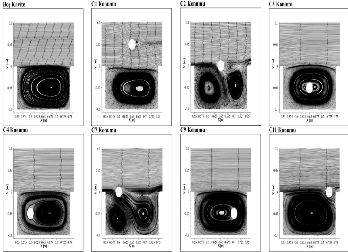
Şekil 7. Değişen silindir konumlarına göre kavite içindeki akım çizgileri
