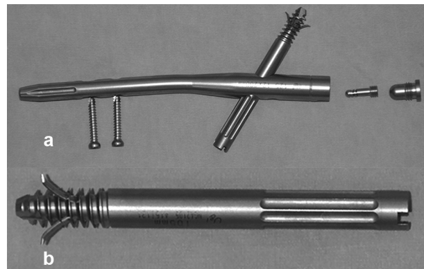
Şekil 1 (a,b): a) DLT™ çivisinin görüntüsü, b) kama kanatlı boyun vidasının (antirotasyon) görüntüsü.
