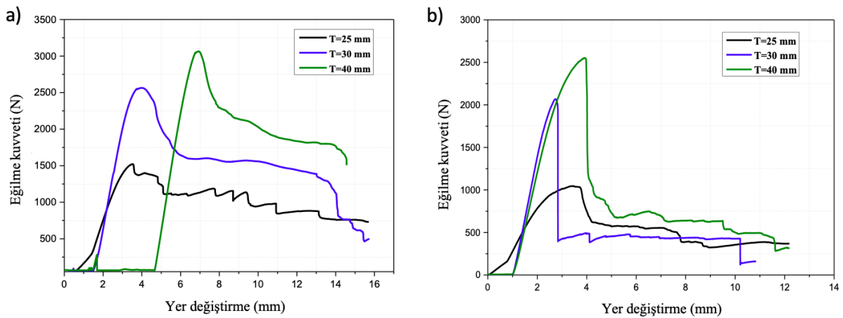
Şekil 5. H = 7 mm hücre boyutuna sahip a) PLA, b) ABS termoplastik petek yapılı kompozit levhaların üç nokta eğilme deneyi sonrası eğilme kuvveti-yer değiştirme grafiği
