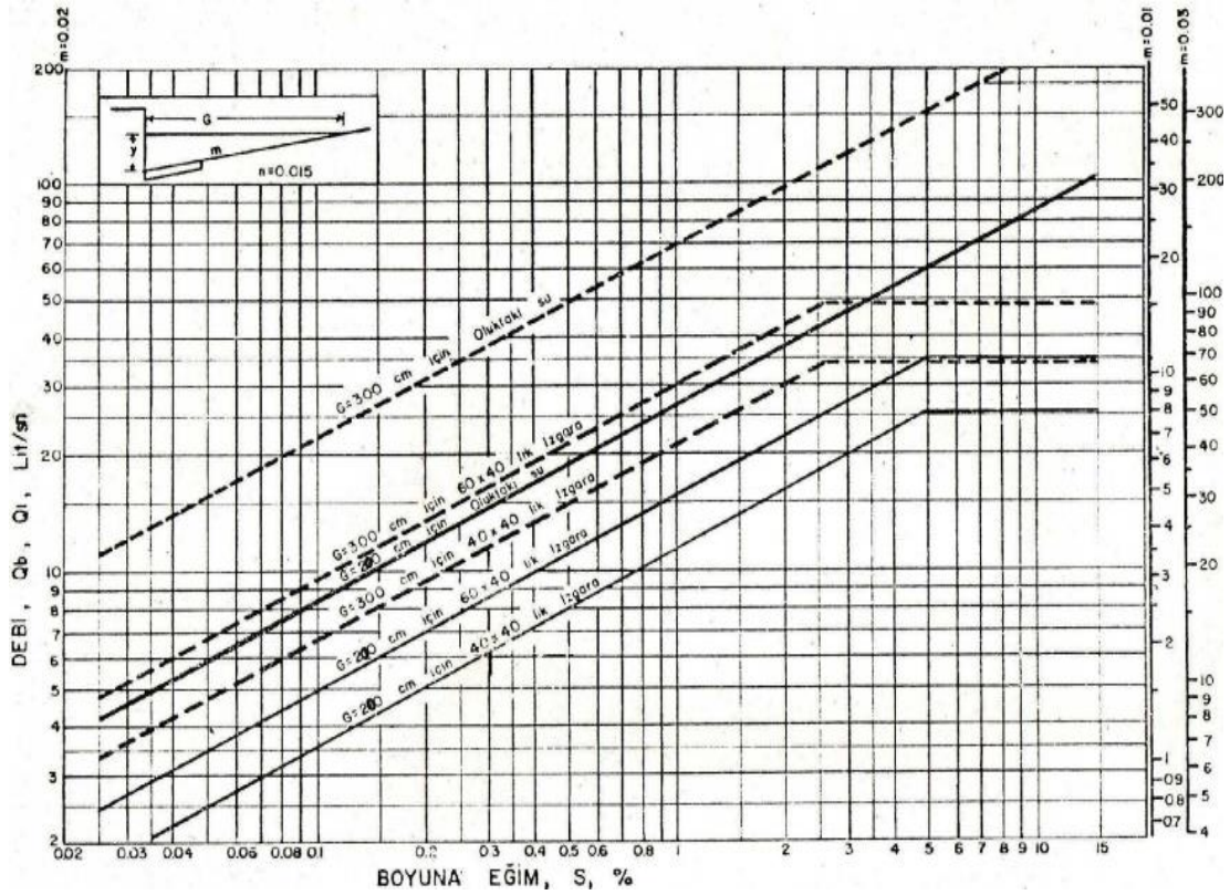
Şekil 7. G=200 cm ve G=300 cm'ye göre bordür oluğu su kapasitesi ve 60x40 ile 40x40 T.C.K'nın tip ızgaralarının su alma kapasiteleri [18].
