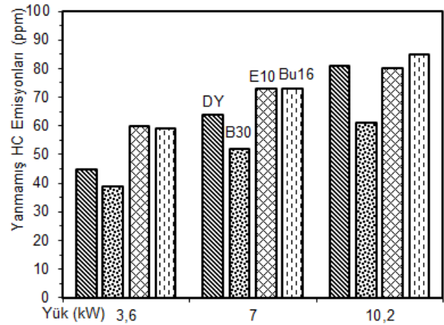
Şekil 5. Deney yakıtlarının HC değerlerinin yük ile değişimi.
