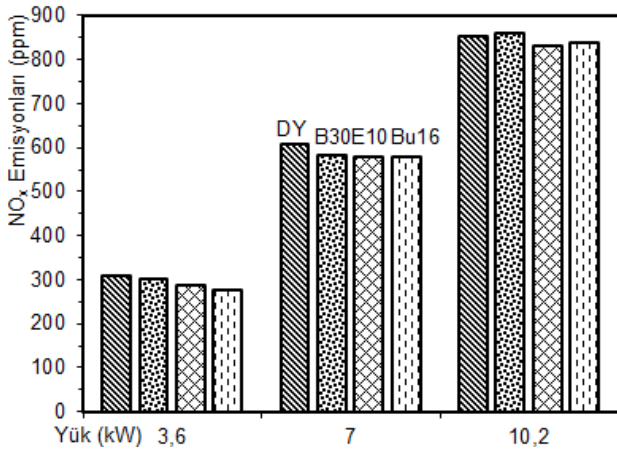
Şekil 4. Deney yakıtlarının \text{NO}_x değerlerinin yük ile değişimi.
