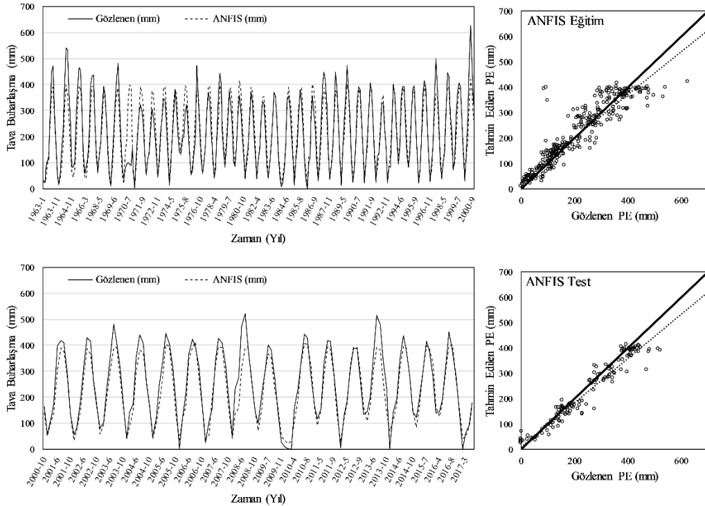
Şekil 6. Diyarbakir istasyonu için gözlenen ve ANFIS yöntemi ile tahmin edilen tava buharlaşma değerlerinin dağılımı
