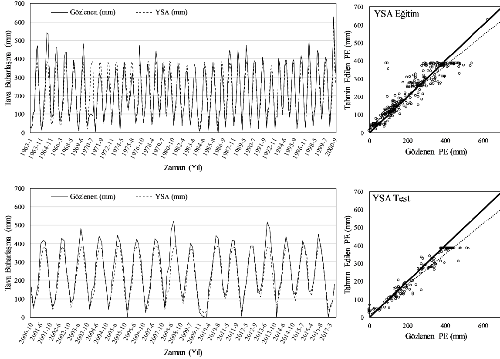
Şekil 5. Diyarbakir istasyonu için gözlenen ve YSA yöntemi ile tahmin edilen tava buharlaşma değerlerinin dağılımı
