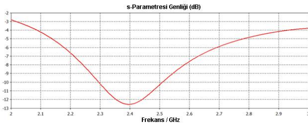
Şekil 2. Dipol anten için dB olarak geri dönüş kaybı grafiği (f=2.4 GHz)
