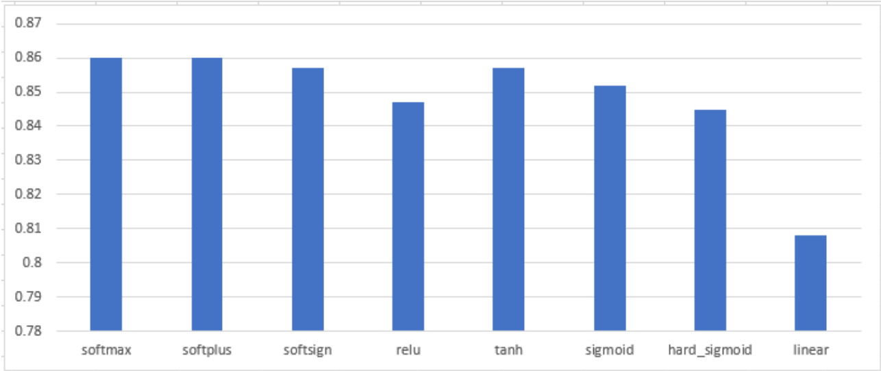
Şekil 7: Aktivasyon Fonksiyonları için Ortalama Doğruluk Sonuç Grafiği
