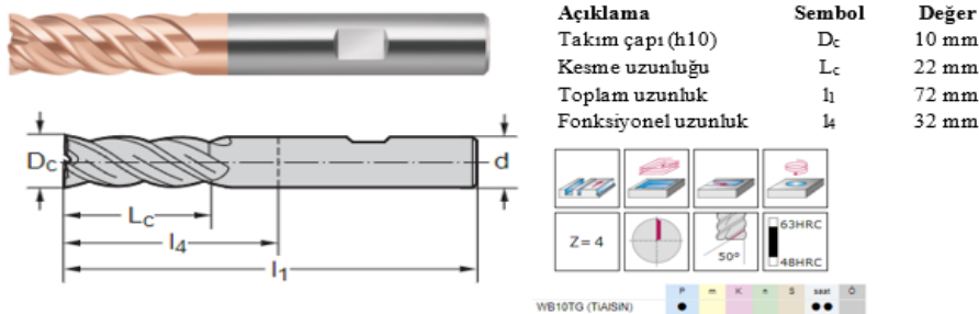
Şekil 1. Deneyisel çalışmalarda kullanılan kesici takım geometrisi.
