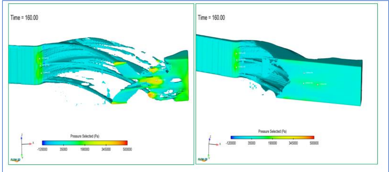
Şekil 27. Hava Sürüklenme Modeli Öncesi ve Sonrası Mansap Kanalı Tabanındaki Basınç Sınıflandırması ( Q12500\text{m}^3/\text{s} Varyant-I)
