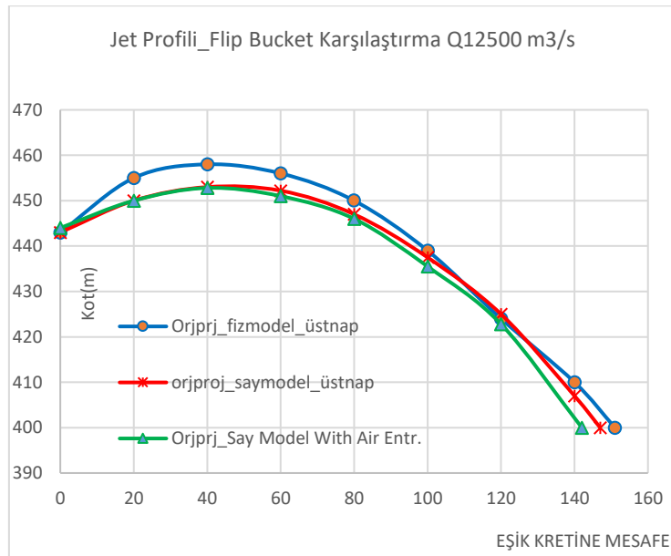
Şekil 25. Flip Bucket Jet profilleri (Q12500 m 3 /s)
