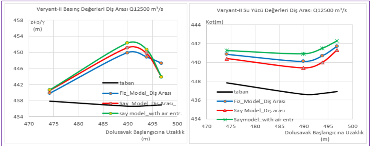
Şekil 21. Varyant-II Diş Arası Basınç ve Su Yüzü Değerleri
