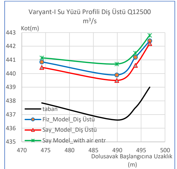
Şekil 18. Varyant-I Diş Üstü Su yüzü Değerleri
