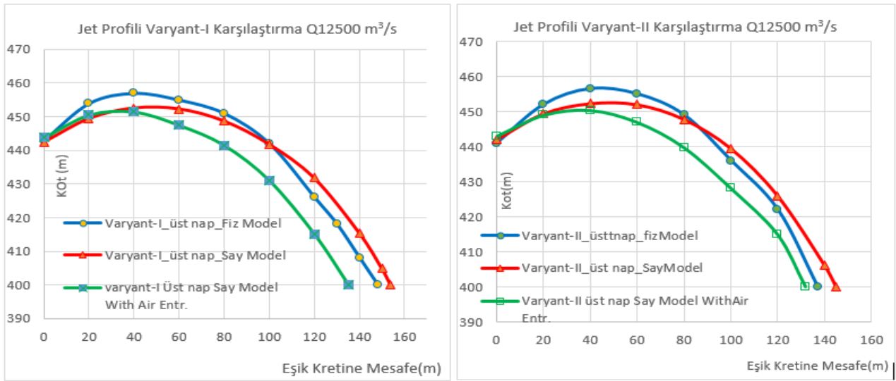
Şekil 24. Varyant-I ve Varyant-II Jet profilleri (Q12500 m 3 /s)
