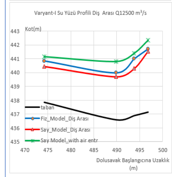
Şekil 19. Varyant-I Diş Arası Basınç ve Su Yüzü Değerleri
