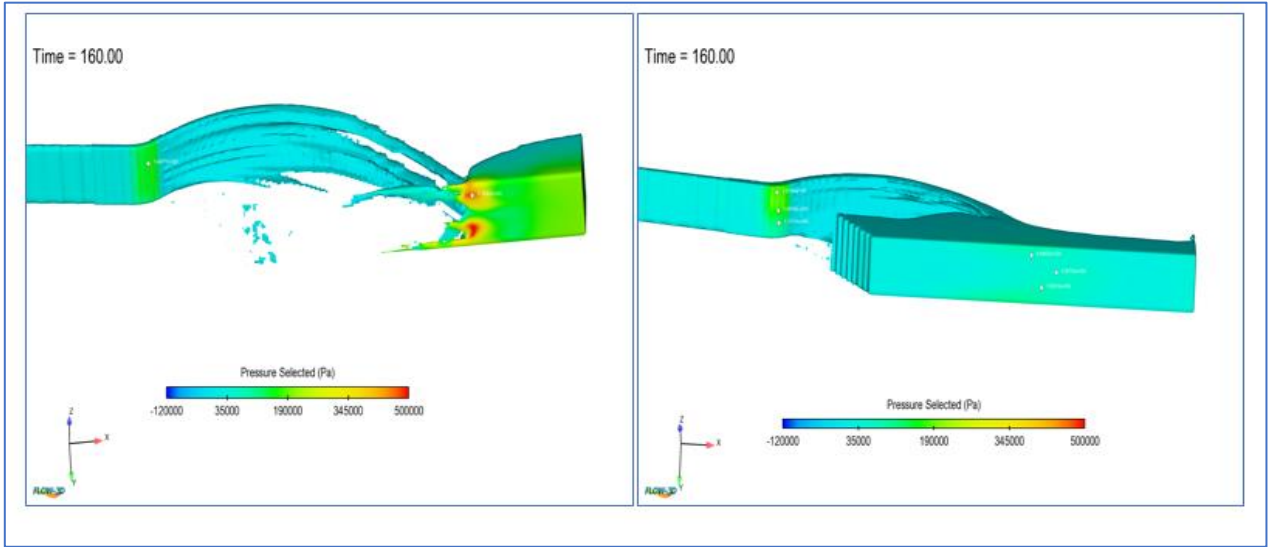
Şekil 26. Hava Sürüklenme Modeli Öncesi ve Sonrası Mansap Kanalı Tabanındaki Basınç Sınıflandırması ( Q12500\text{m}^3/\text{s} Flip Bucket)
