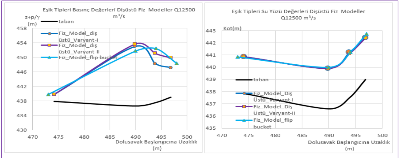
Şekil 23. Sıçratma Eşik Tipleri Basınç ve Su Yüzü Değerleri Fiziksel Modeller
