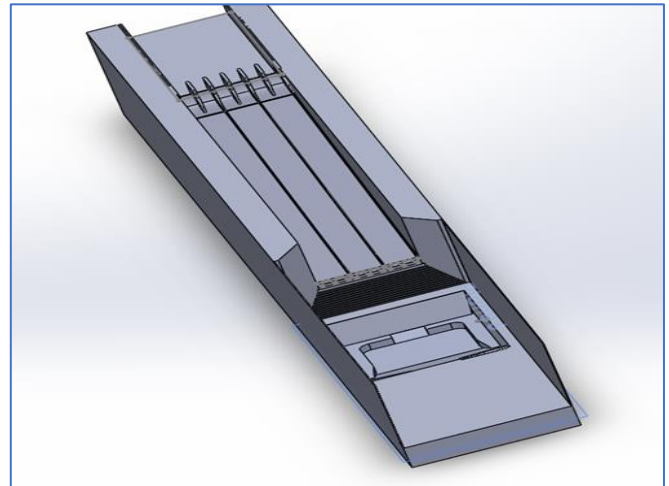
Şekil 6. Ilısu Barajı 2010 Yılı Dolusavak 3D Yapısı
