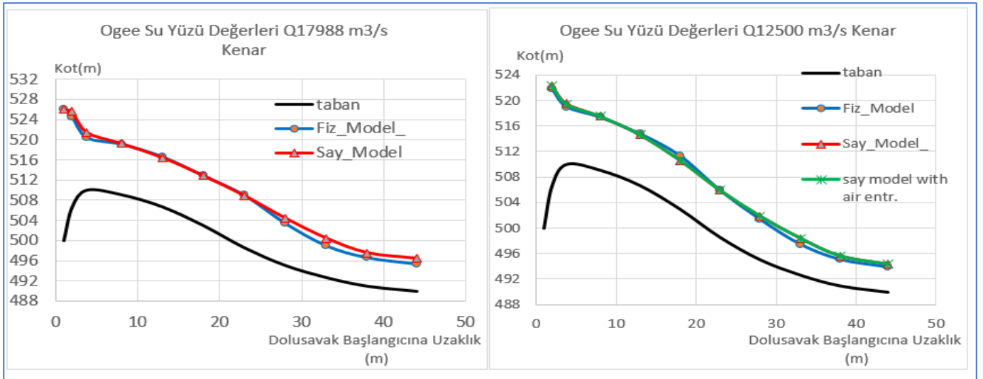
Şekil 13. a. Su Yüzü Değerleri Ogee Eksen (Q17988 m 3 /s) b. Su Yüzü Değerleri Ogee Kenar (Q12500 m 3 /s)
