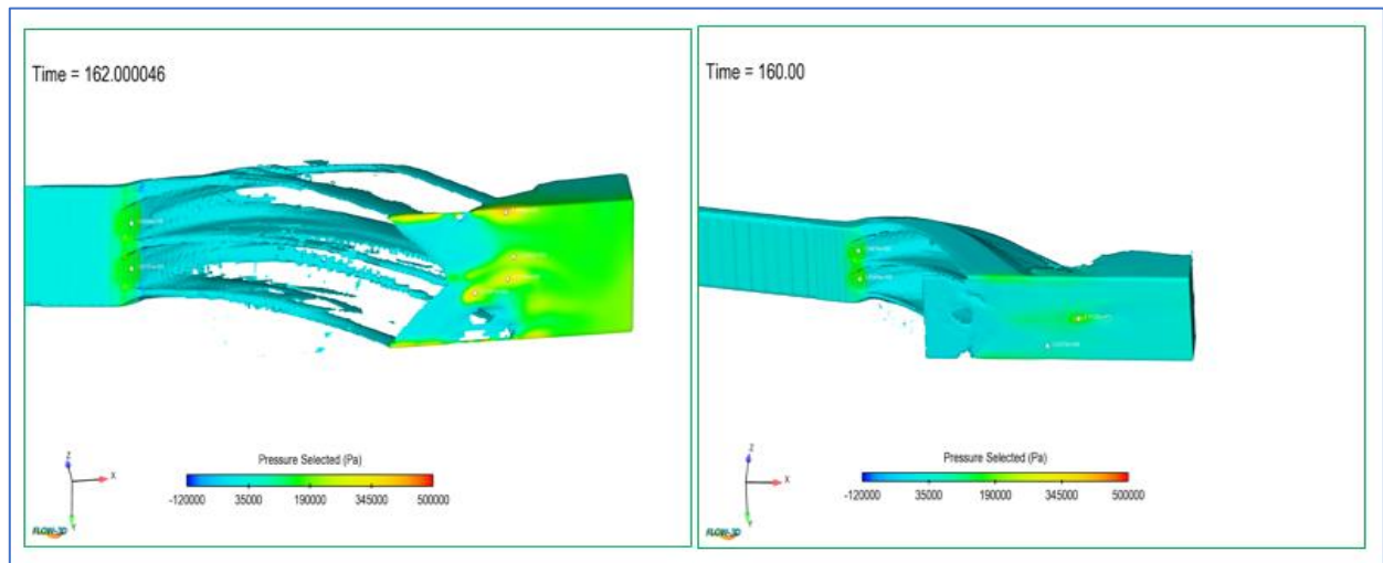
Şekil 28. Hava Sürüklenme Modeli Öncesi ve Sonrası Mansap Kanalı Tabanındaki Basınç Sınıflandırması ( Q12500\text{m}^3/\text{s} Varyant-II)
