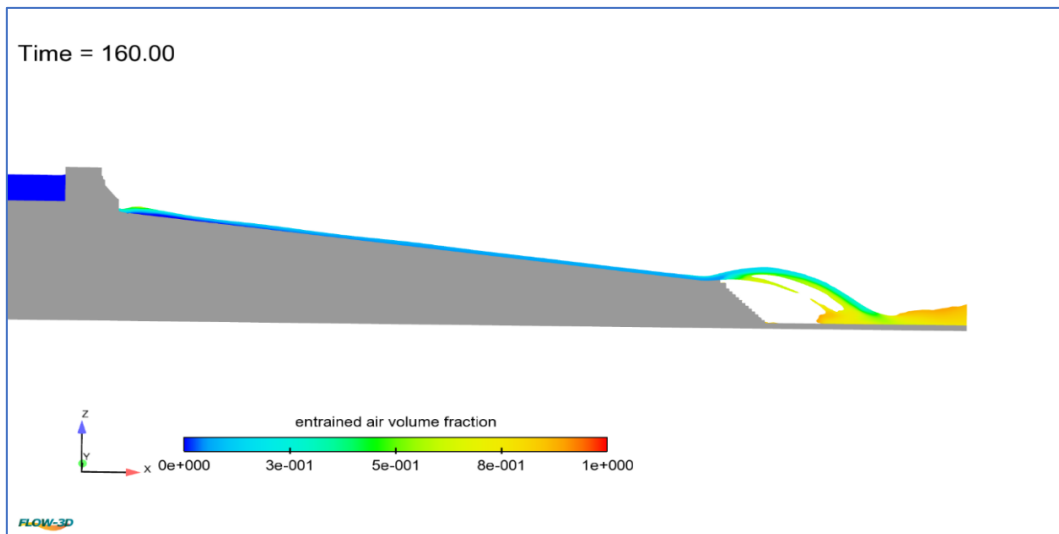
Şekil 14. Dolusavak Akıma Giren Hava Değerlerine Göre Sınıflandırma ve 2D Eksen Kesiti (Q12500 m 3 /s)
