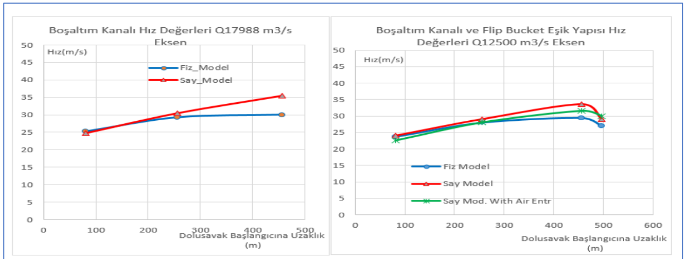
Şekil 16. a. Boşaltım Kanalı Hız Değerleri 17988 m³/s b. Boşaltım Kanalı ve Flip Bucket Hız Değerleri (Q12500m³/s)
