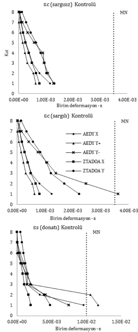
Şekil 10. Çekirdek U perde için kesit bazında performans değerlendirmesi
