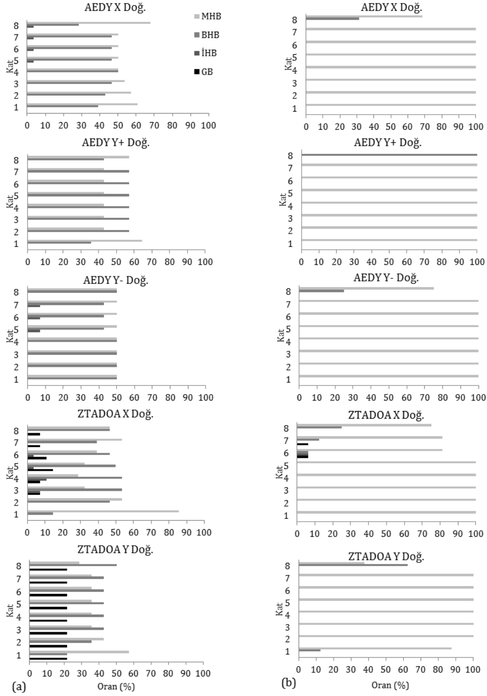
Şekil 9. Eleman bazında performans seviyeleri: (a) kirişler, (b) kolonlar
