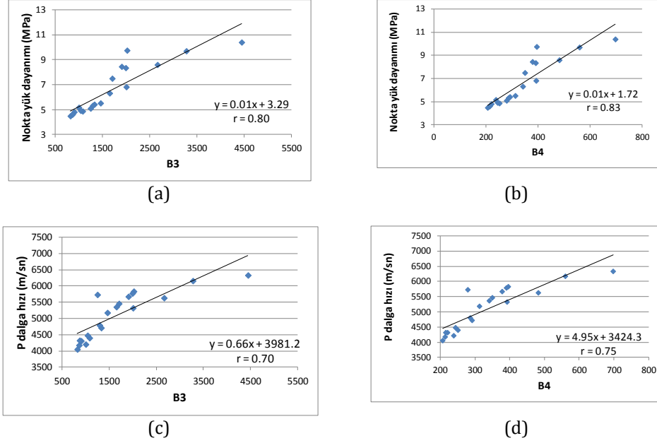
Şekil 2. Mağmatik kayaçlar için, nokta yük dayanımı ve P dalgası hızı ile B3-B4 kırılabilirlik indeksleri arasındaki ilişki a) nokta yük dayanımı ile B3 arasındaki ilişki, b) nokta yük dayanımı ile B4 arasındaki ilişki, c) P dalgası hızı ile B3 arasındaki ilişki, d) P dalgası hızı ile B4 arasındaki ilişki.
