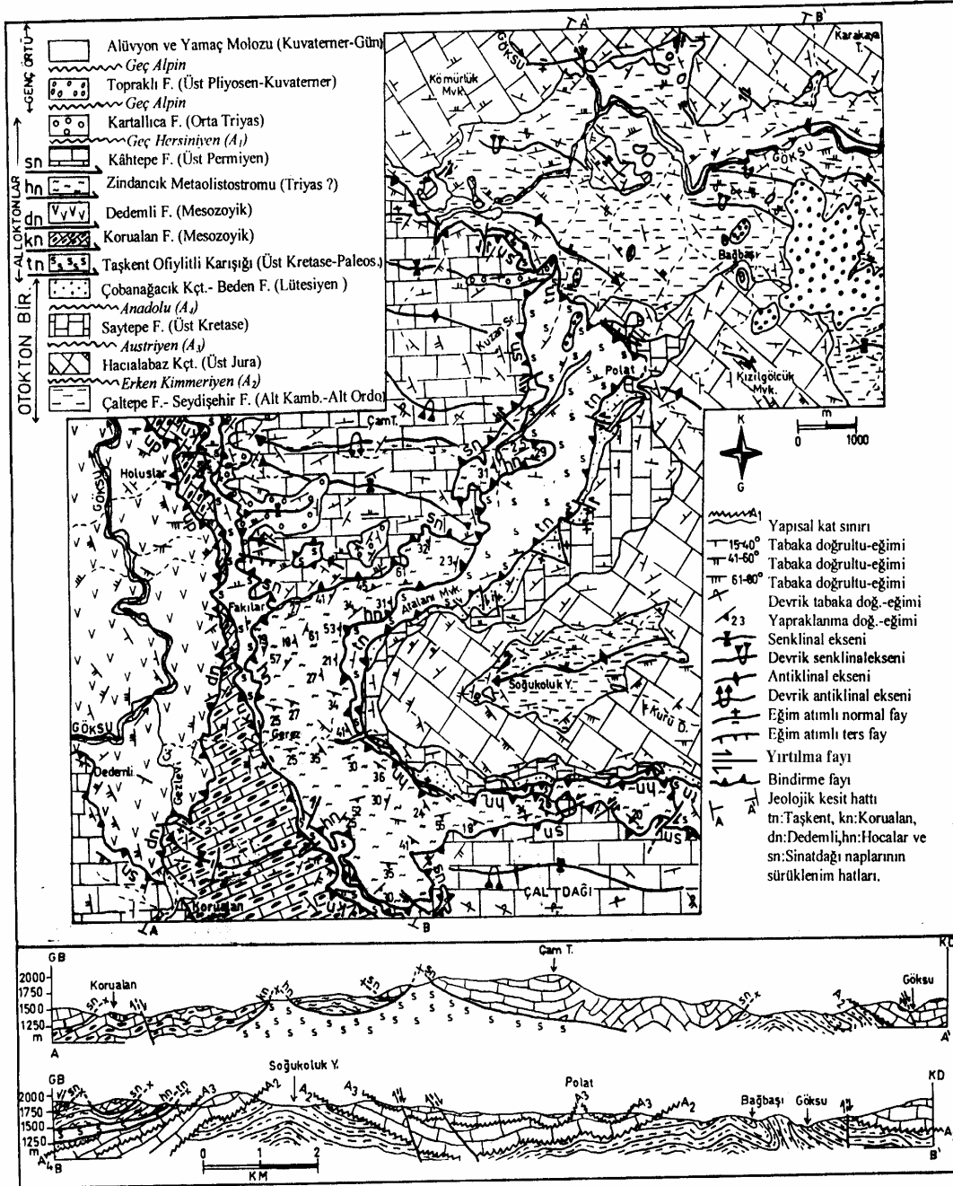
Şekil 3. İnceleme alanının yapısal haritası ve kesitleri
