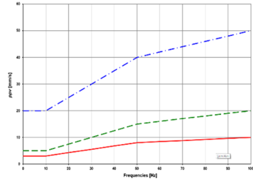
Şekil 3. Alman DIN4150 Hasar Kriteri
