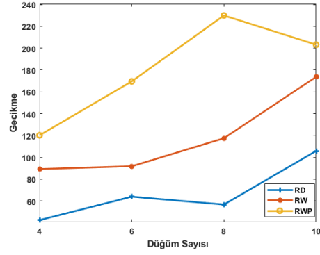
Şekil 10. 300x300 alan için mesaj iletme gecikmesi
