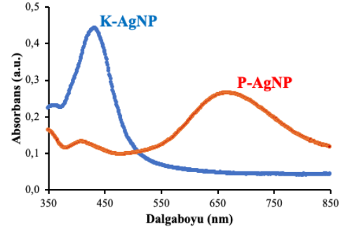
Şekil 1. Küresel (K-AgNP, mavi) ve prizmatik (P-AgNP, turuncu) nanogümüşe ait UV-Vis-NIR spektrumları
