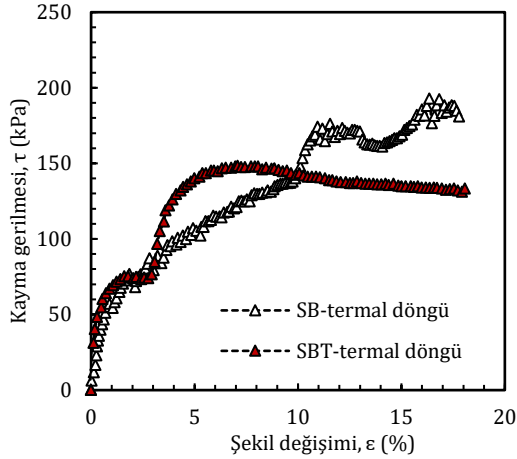
Şekil 4. Tinkal katkılı kum-bentonit karışımlarının termal döngü altında kayma gerilmesi-şekil değişimi grafiği
