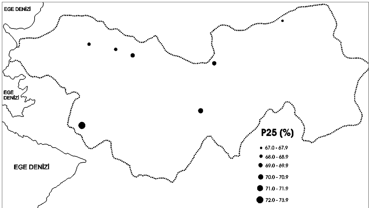
Şekil 4. Yağışlı günlerin en yüksek kuartilinin sağladığı yağışın toplam yağış içindeki yüzdesinin (P25) havzadaki konumsal değişimi.
