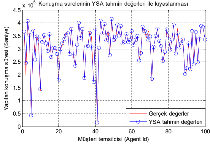
Şekil 5. Gelen Çağrılarının Görüşme Sürelerinin Gerçek Değerleri ve YSA Tahmin Değerleri
