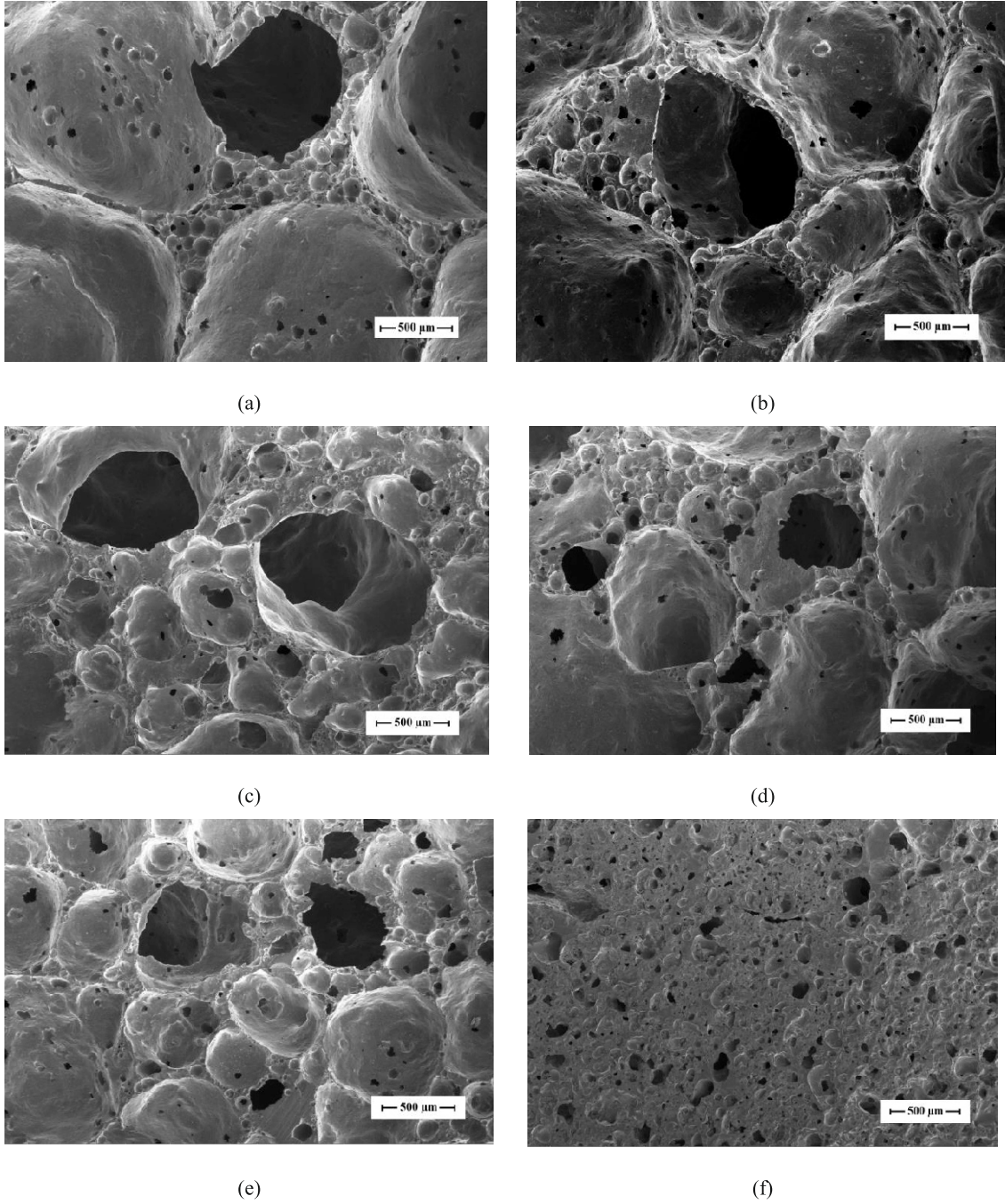
Şekil 3. Farklı \text{Al}_2\text{O}_3 oranları ile hazırlanan cam köpük malzemelerin SEM görüntüleri; a) A0, b) A1, c) A5, d) A10, e) A20, f) A40.
