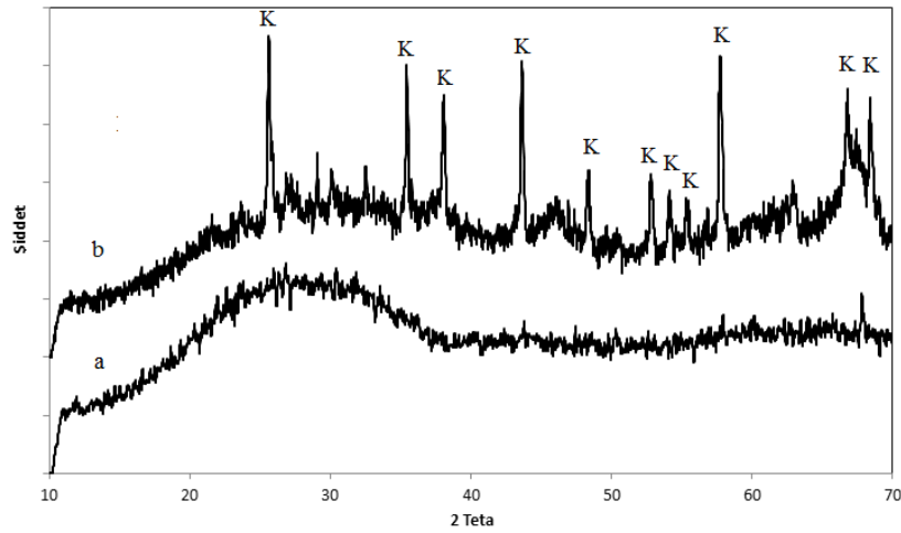
Şekil 4. Alümina katkısız ve %20 alümina katkılı cam köpük malzemelerin faz analizleri: a) alümina katkısız, b) %20 alümina katkılı, K: korundum fazı
