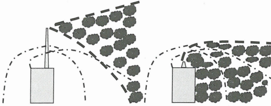
Şekil 3. Baca Konumuna Göre Duman Hareketleri[7]
