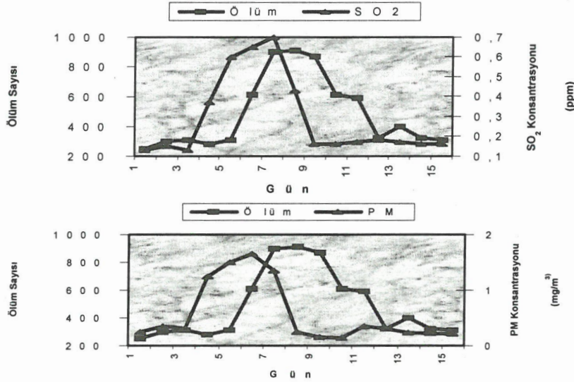
Şekil 4. 1952 Londra Episodunda Meydana Gelen Ölüm ve SO 2 ve PM Konsantrasyonları[10]
