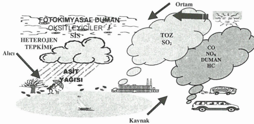
Şekil 2. Hava Kirleticilerin Oluşum Mekanizması[6]
