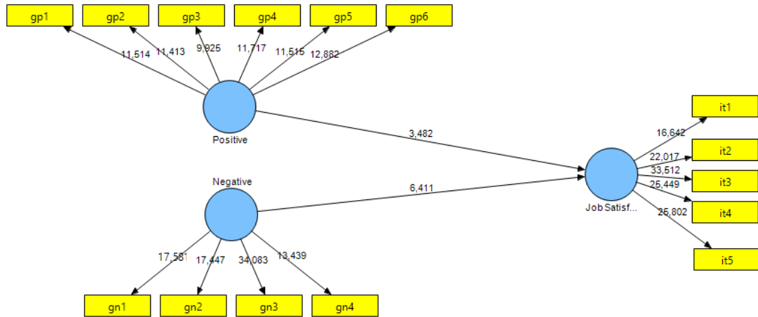
Şekil 2: Modele İlişkin t Değerleri
