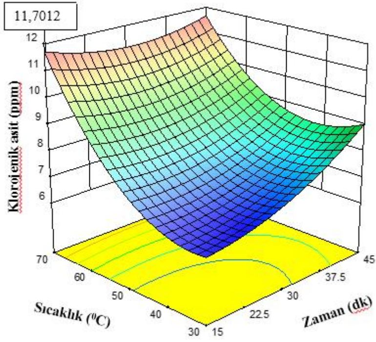
Şekil 5. Ekstraksiyon sıcaklığına zaman oranının bir fonksiyonu olarak dişbudak ağacı yapraklarından klorojenik asit verimi için yüzey yanıt grafiğı
