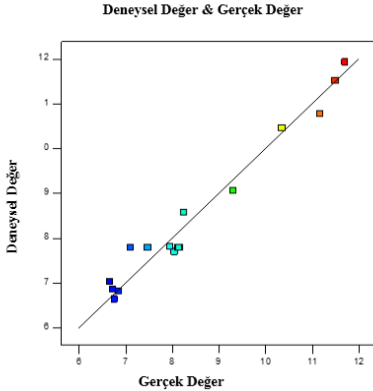
Şekil 8. Dişbudak yaprağı için denklemden elde edilen değerler ile deneysel verilerin karşılaştırılması (Deneyisel veriler Tablo 4 te verilmiştir)
