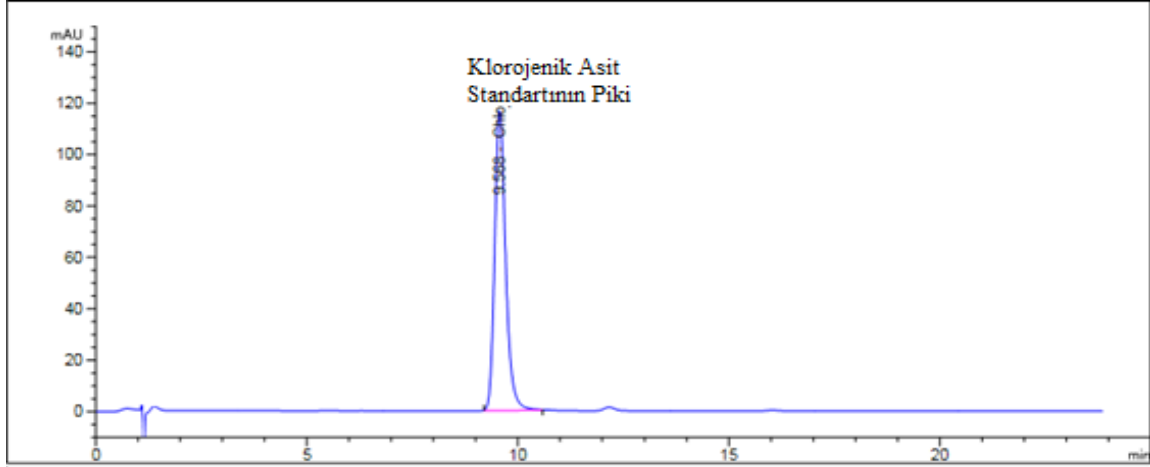
Şekil 9. Klorojenik asit standardının kromatogramı
