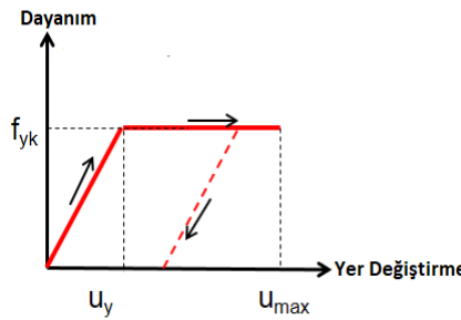
Şekil 1. Sünek davranışa ait dayanım-yer değiştirme grafiği
