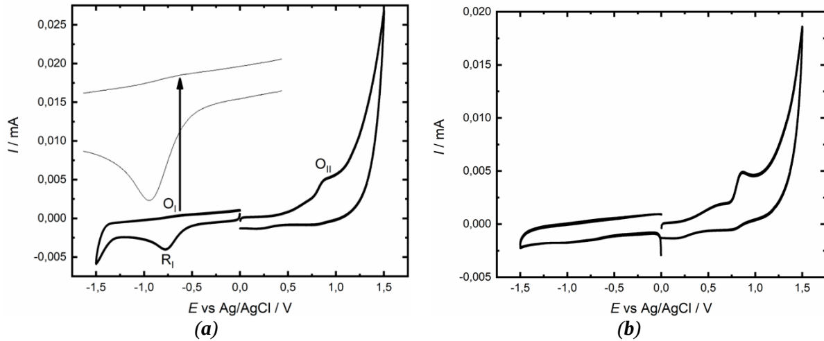
Şekil 9. 1 mM’lık ZnLCl 2 ’nin (a) ve L’nin (b) argon gazı ile doyurulmuş 0.1 M TBATFB içeren bir DMF çözeltisi içerisindeki camı karbon elektrot yüzeyinde 100 mV s -1 tarama hızında kaydedilen CV’si.
