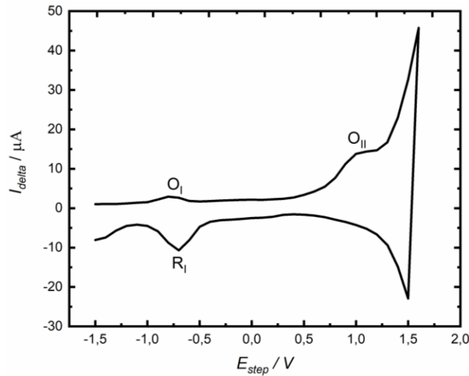
Şekil 10. 1 mM ZnLCl_2 'nin argon gazı ile doyurulmuş 0.1 M TBATFB içeren bir DMF içerisindeki camı karbon elektrot yüzeyinde 100 \text{ mV s}^{-1} tarama hızında kaydedilen SWV'si.
