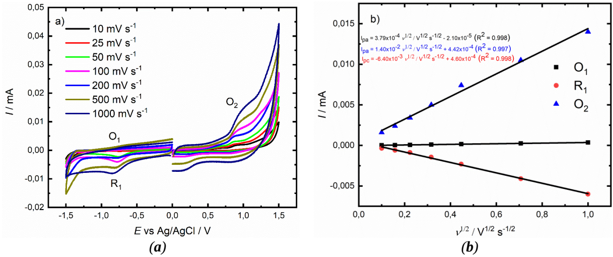
Şekil 11. (a) 1 mM ZnLCl 2 kompleksinin argon gazı ile doyurulmuş 0.1 M TBATFB içeren bir DMF içerisindeki camı karbon elektrot yüzeyinde farklı tarama hızında kaydedilen CV'leri. (b) anodik ve katotik pik akımının tarama hızının karekökü ile lineer ilişkisini göstermektedir.
