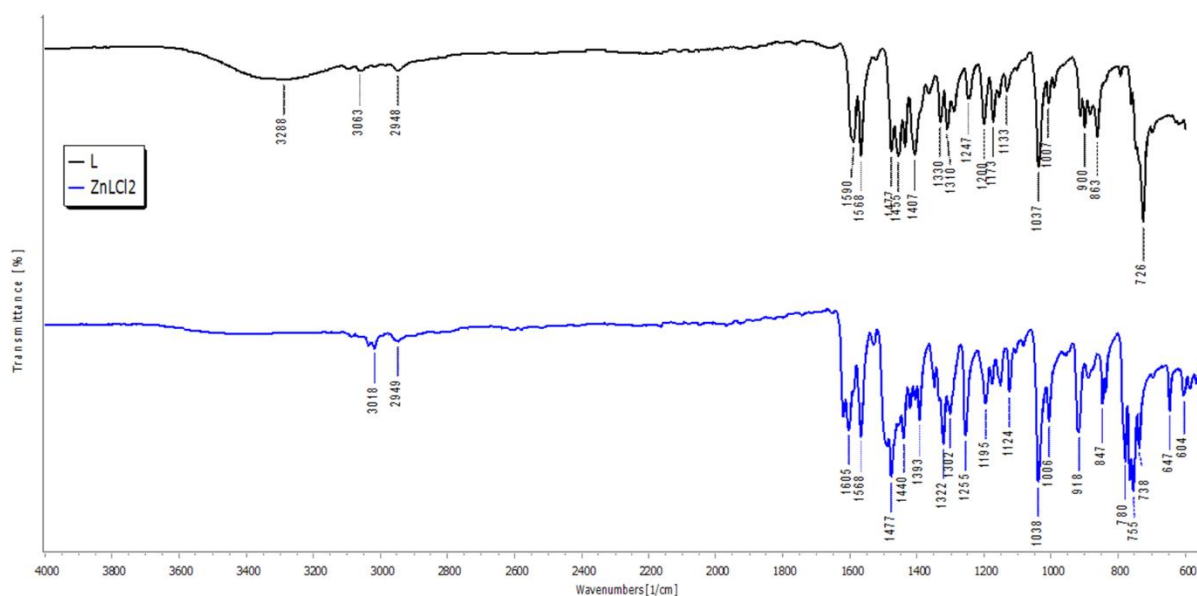
Şekil 3. L ve ZnLCl 2 moleküllerine ait FT-IR spektrumları.
