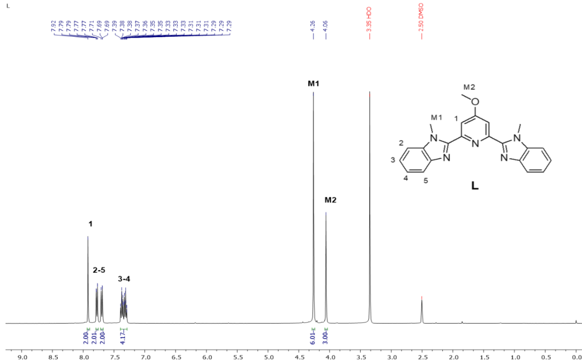
Şekil 5. L molekülünün ^1\text{H} NMR spektrumu.
