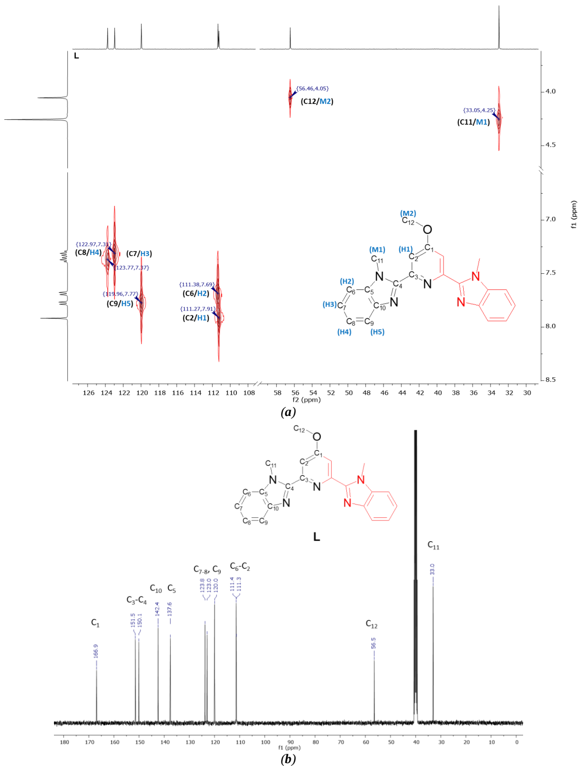
Şekil 6. L molekülünün HETCOR (a) ve ^{13}\text{C} NMR (b) spektrumları.
