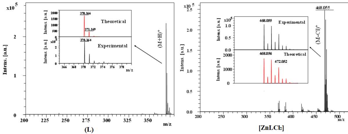
Şekil 4. L ve \text{ZnLCl}_2 moleküllerine ait MALDI-TOF-MS spektrumları.
