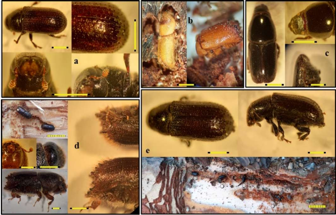
Şekil 3. Tespit edilen türlerden Tomiscus minor (a), Orthotomicus erosus (b), Scolytus mali (c), Ips sexdentatus (d), Tomiscus piniperda (e) (1 mm)
