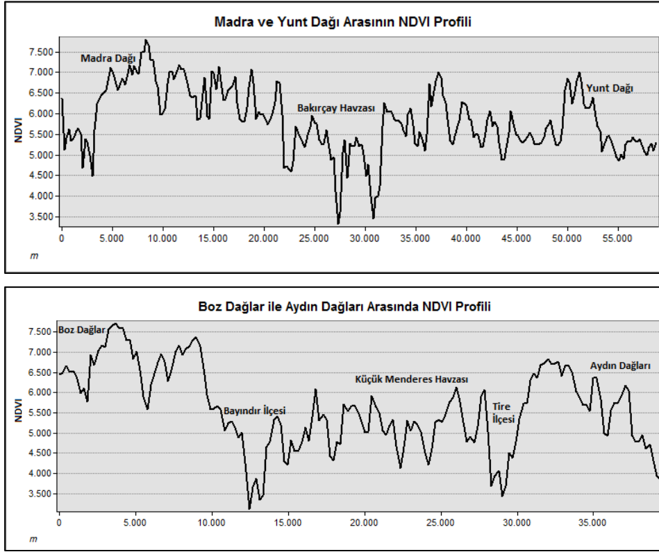
Şekil 5. Ege Bölgesinin bazı horst ve graben sistemlerinde NDVI profili (2012 yılının ocak ayına ait veri).
