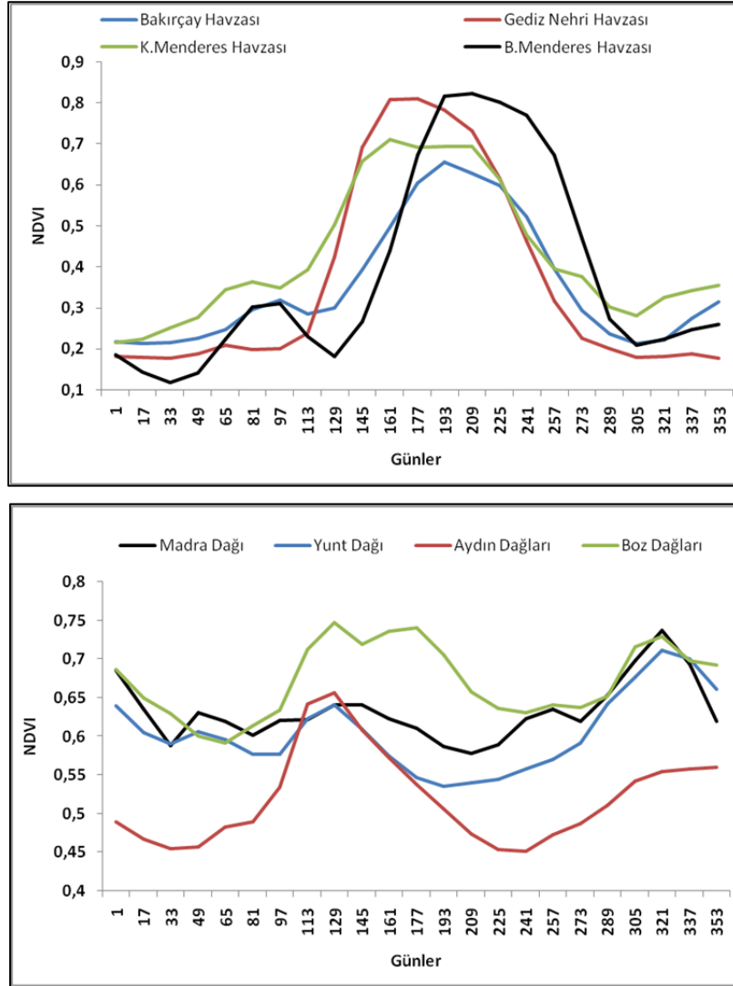
Şekil 6. Ege Bölgesi'ndeki belli başlı zonobiom (üstte) ve orobiom (altta) alanlarında NDVI değerleri.
