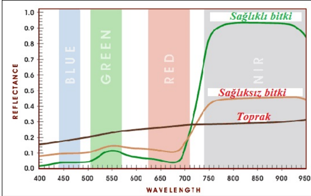
Şekil 2. Vegetasyonun yakın infrared radyasyona verdiği tepki. (kaynak: http://agrielectronics.blogspot.com.tr/2013_10_01_archive.html?*=1 ).
