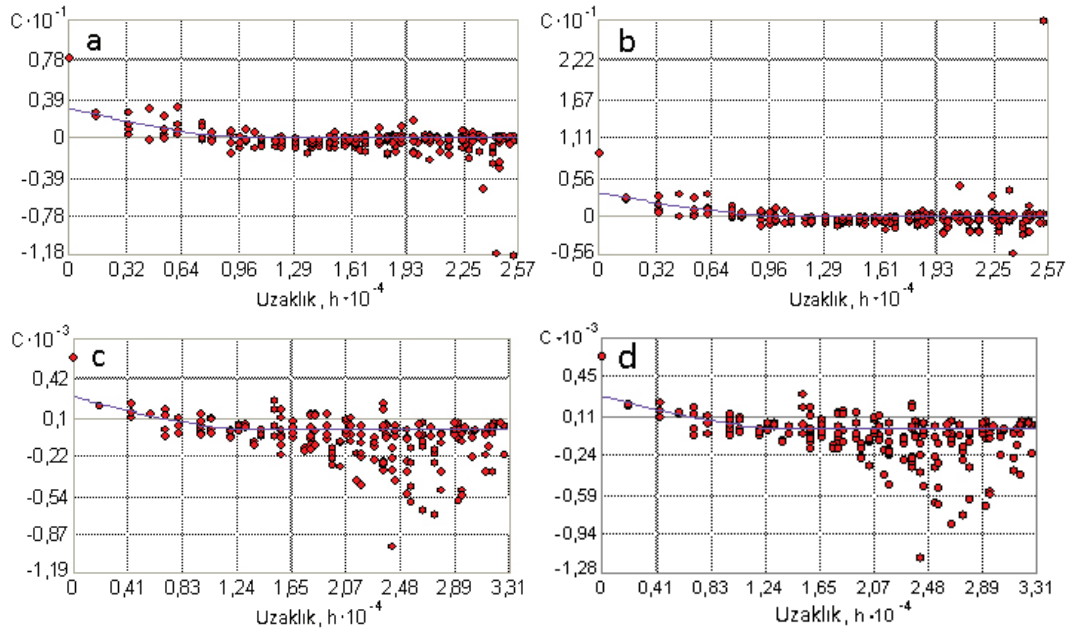
Şekil 4: Kovaryans grafikleri. a) 0-20 cm derinlik organik madde, b) 20-40 cm derinlik organik madde, c) 0-20 cm derinlik KDK, d) 20-40 cm derinlik KDK
