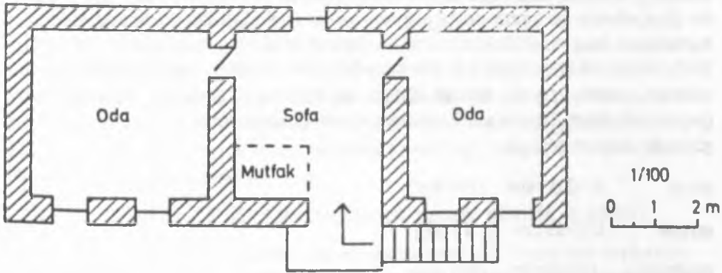
Şekil 3.a- Gökeyüp köyünde eskiden kalma, günümüzde kullanılmayan düz toprak damlı konuta ait bir plan (konut iki katlı olup, plan 2.kata aittir, alt kat ahırdır, tuvalet avlunun bir köşesindedir).
