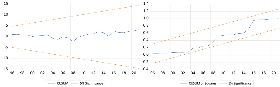
Şekil 3: CUSUM Grafikleri
