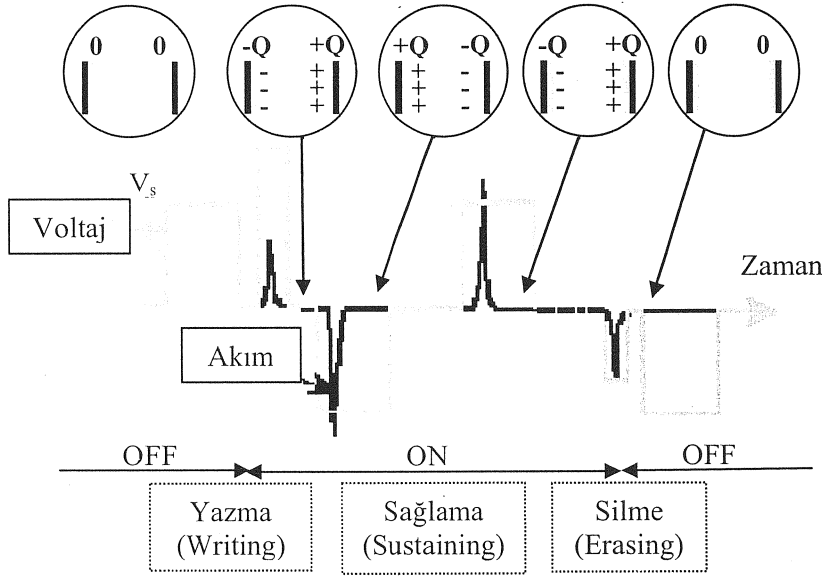
Şekil 1. PPE'nin akım ve voltaj pulsaları.
