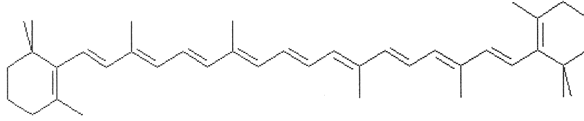
Şekil 1. Beta karoten'nin moleküler yapısı
