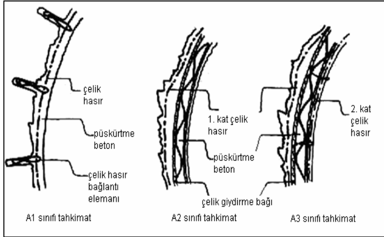
Şekil 2. Tahkimat çeşitleri [6].
