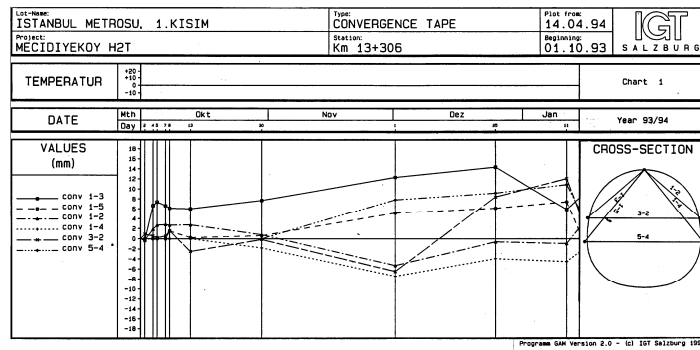
Şekil 7. 13306. metrede yapılan konverjans ölçümü (mm) [17].
