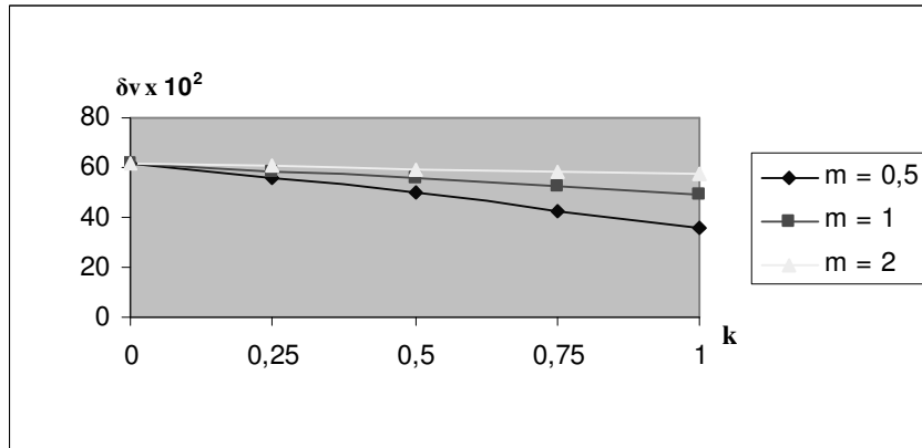
Şekil 2. \frac{T_0 \alpha_0}{h} = 2 için ' k ' parametresine bağlı olarak düşey yer değiştirmelerin gösterimi
