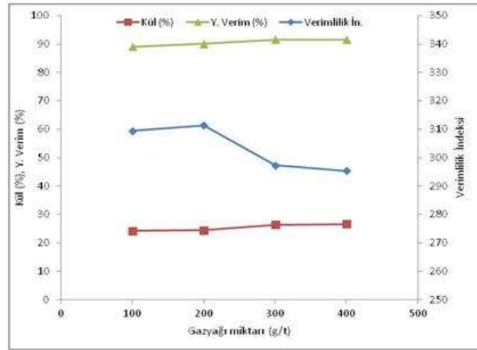
Şekil 3. En uygun gazyağı miktarı için yapılan deney sonuçları (Oktanöl: 75 g/t, devir: 1400 dev/dk, katı oranı : %11)
