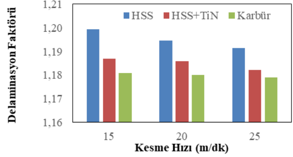
Şekil 6. 0.05 mm/dev ilerleme hızında oluşan delaminasyon faktörü
