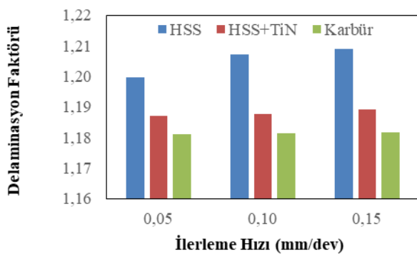
Şekil 9. 15 m/dk kesme hızındaki oluşan delaminasyon faktörü
