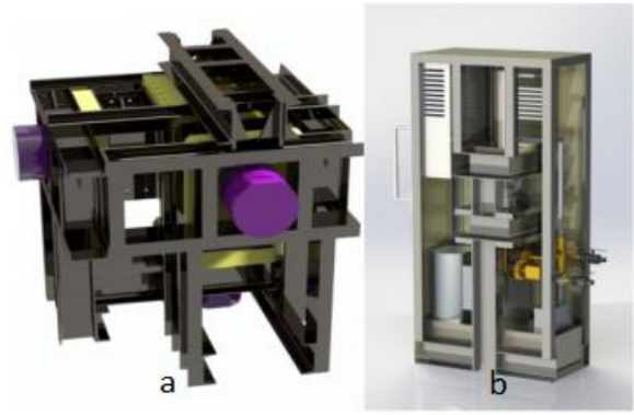
Şekil 2. a) Gerçek üç eksenli sıkıştırma hücresi b) Hidrolik şırınga pompa modelleri.
