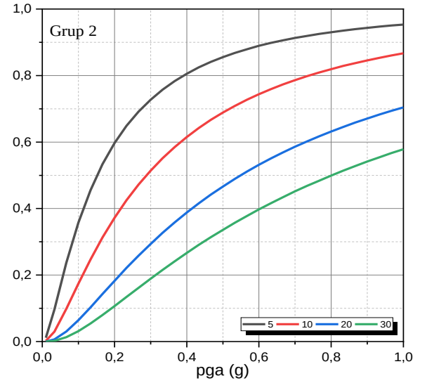
Şekil.15 Kullanılan Kırılgenlik Eğrisi
