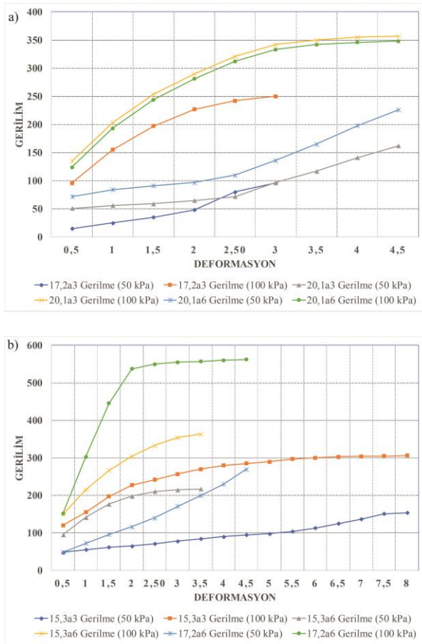
Şekil 7. Düşük plastisiteli (CL) ve yüksek plastisiteli (CH) zemin sınıfına ait numunelerin gerilme deformasyon grafikleri a-) CH zemin sınıfı b-) CL zemin sınıfı.
