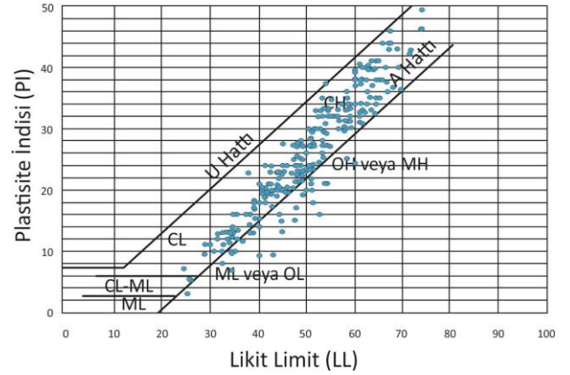
Şekil 6. Casagrande kartı
