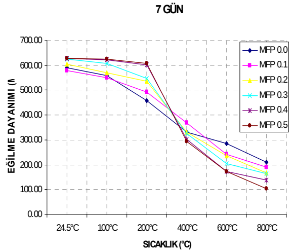
Şekil 7. MFP Lifli 7 Günlük Prizmatik Kırış Numunelerin Eğilme Dayanımı-Sıcaklık Değişimi
