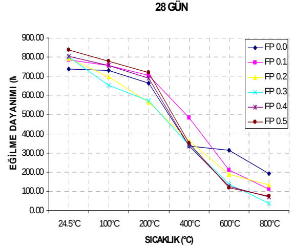
Şekil 5. FP Lifli 28 Günlük Prizmatik Kiriş Numunelerin Eğilme Dayanımı-Sıcaklık Değişimi
