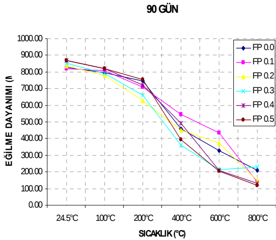
Şekil 6. FP Lifli 90 Günlük Prizmatik Kırış Numunelerin Eğilme Dayanımı-Sıcaklık Değişimi
