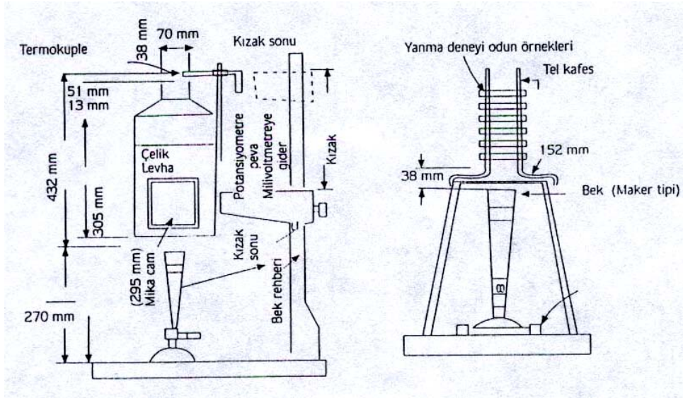
Şekil 2. Yanma Deneyi Düzenegi
